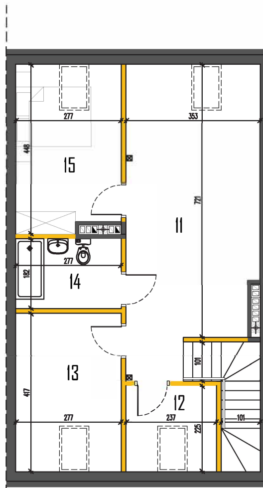
RZUT PODDASZA
